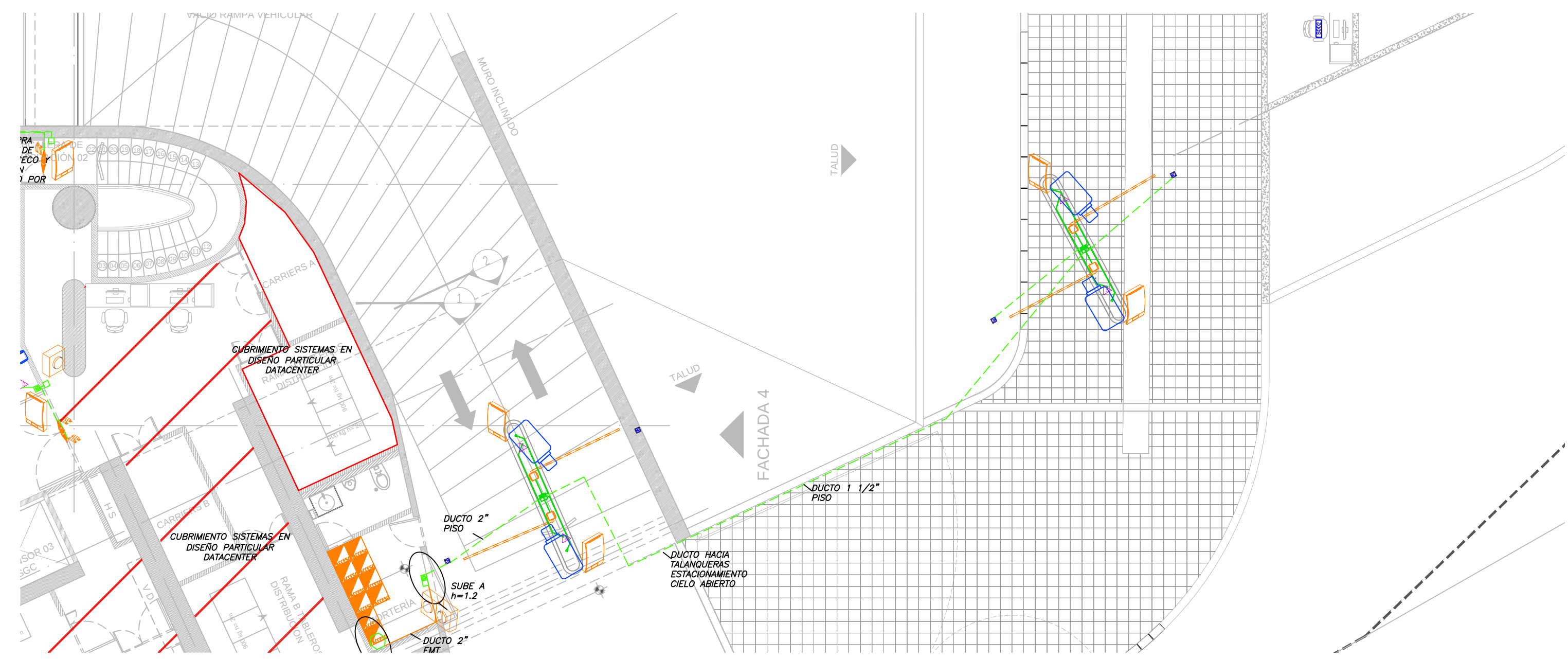
DETALLE TALANQUERA VEHICULAR ESTACIONAMIENTO CIELO ABIERTO
